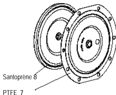
Vue des 2 pièces de la membrane PTFE
